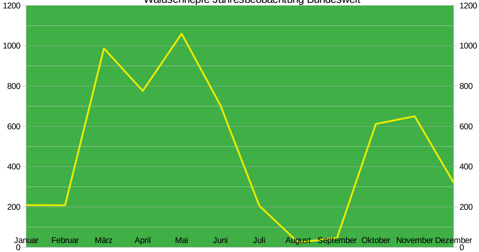
Waldschnepe Jahresbeobachtung Bundesweit
