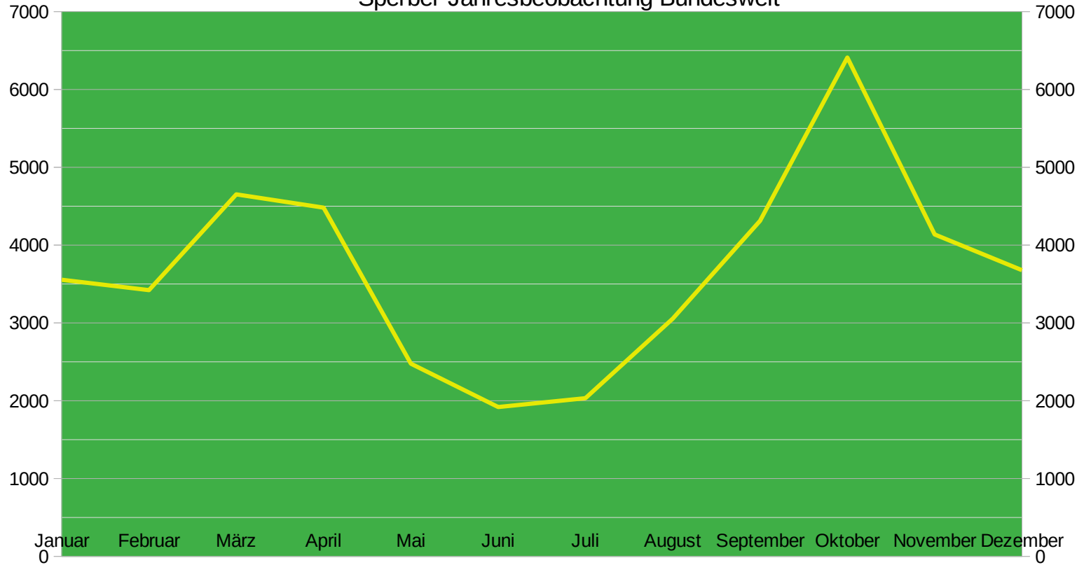
Sperber Jahresbeobachtung Bundesweit
